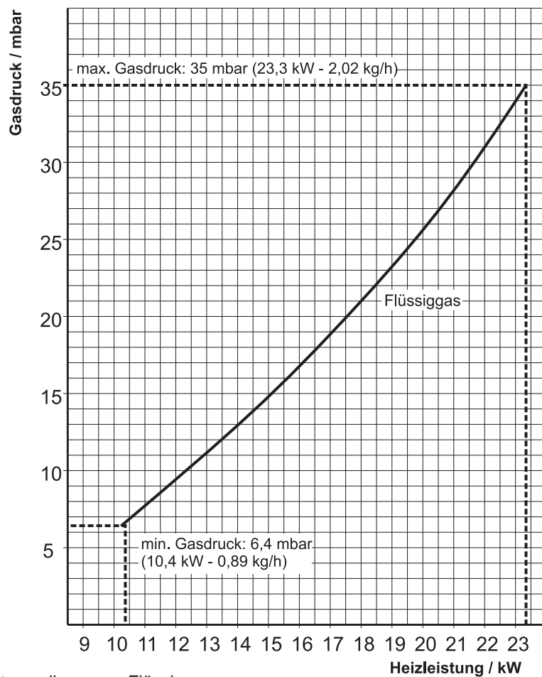
Abb. 5.10 Gas-Leistungsdiagramm Flüssiggas
