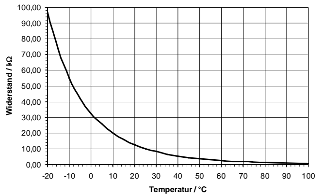
Abb. 4.12 Widerstandskurve
