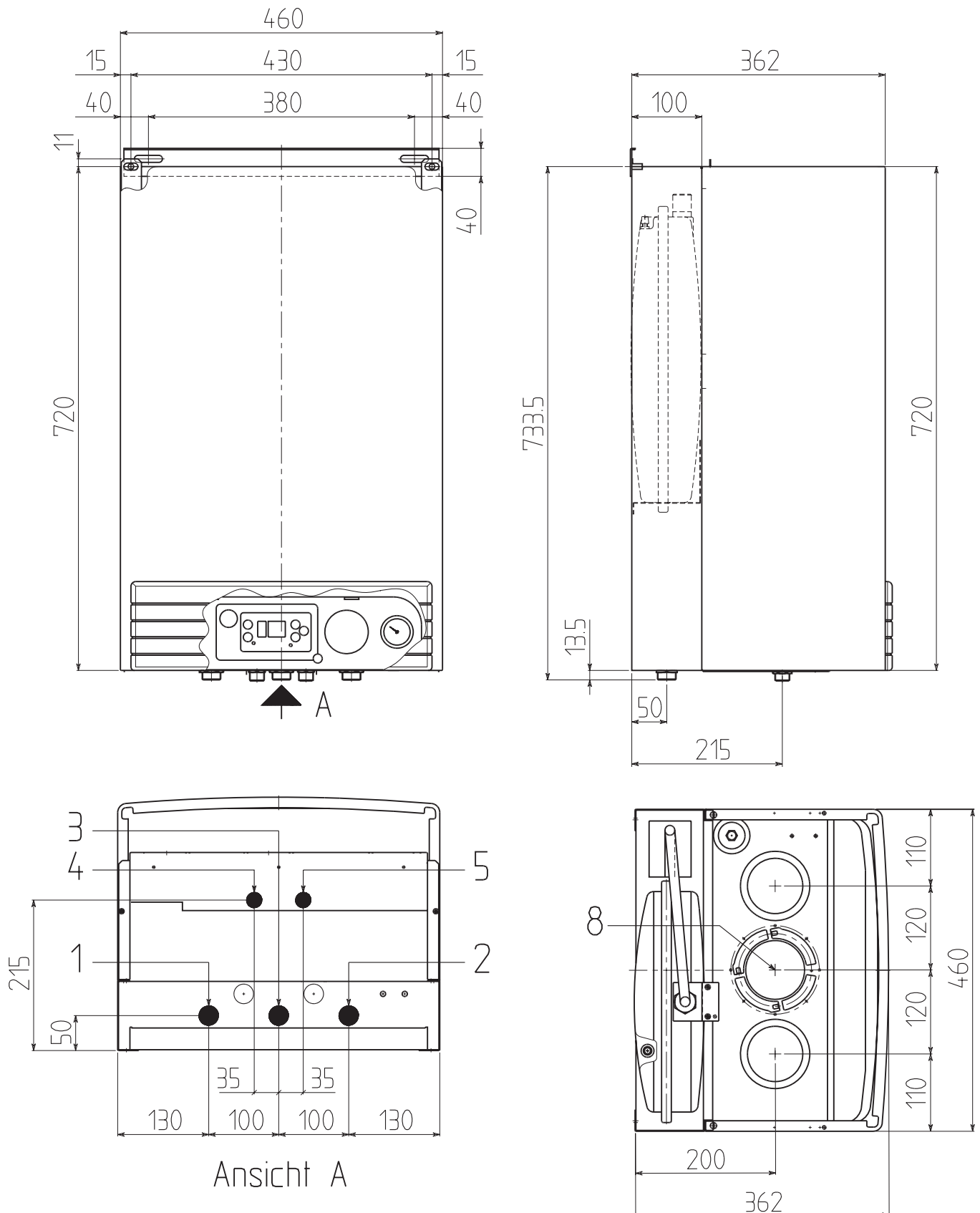
Abb. 2.2 Geräteabmessungen Econtherm CT
