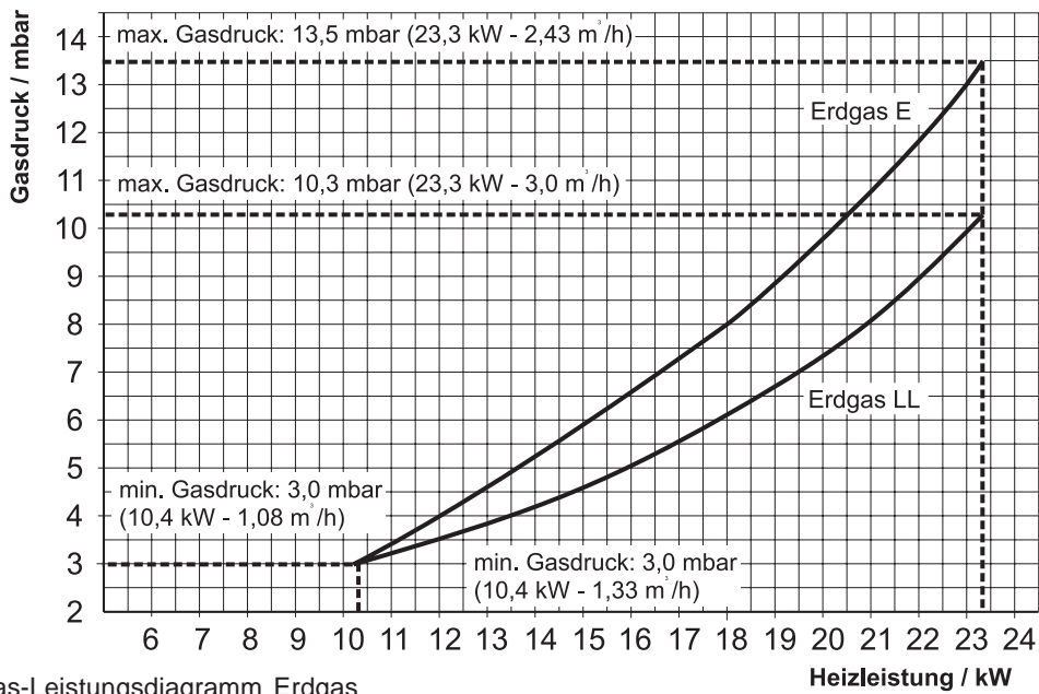
Abb. 5.9 Gas-Leistungsdiagramm Erdgas
